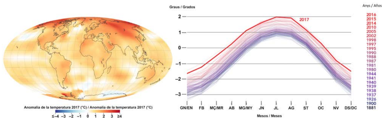
Anomalia de la temperatura (2017 i diferència de la mitjana anual 1881-2017) Anomalía de la temperatura (2017 y diferencia de la media anual 1881-2017)
